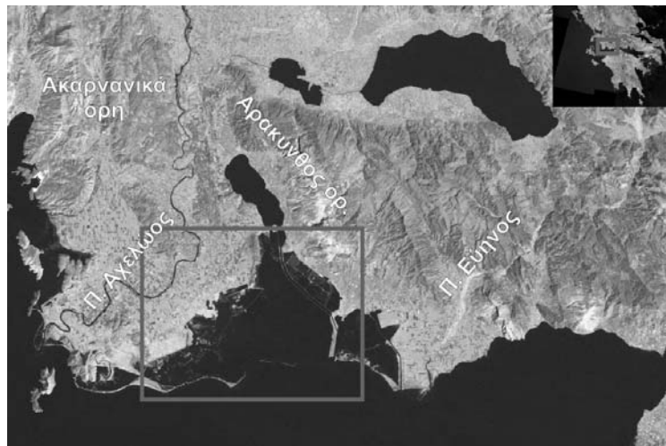
Σχήμα 1. Η περιοχή μελέτης της λιμνοθάλασσας Μεσολογγίου σε ψευδοέγχρωμη δορυφορική εικόνα LANSAT της δεκαετίας του 1990. (Βλέπε έγχρωμο ψηφιακό αρχείο πρακτικών) για χρήση ως χάρτης (NASA, 2003).
