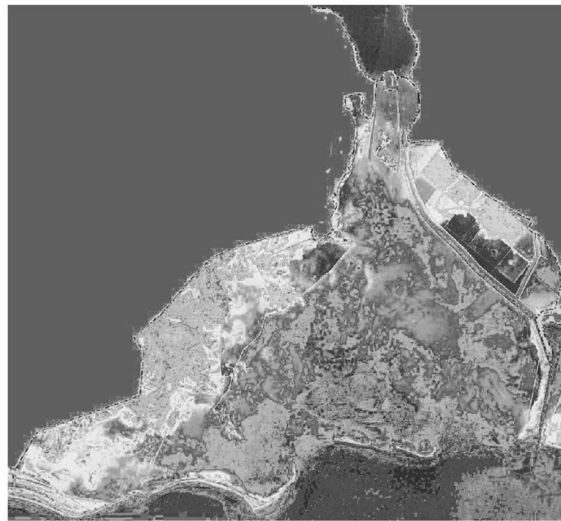
Σχήμα 2. Αριστερά, η διορθωμένη γεωμετρικά δορυφορική φωτογραφία και δεξιά, η ίδια φωτογραφία όπου pixels γνωστό βάθος νερού σε συγκεκριμένες θέσεις ταξινομήθηκαν με ενιαίο χρωματικό τόνο με άλλα pixels τα οποία είχαν συγγενή απόχρωση στην αρχική φωτογραφία. (Βλέπε έγχρωμο ψηφιακό αρχείο πρακτικών).
