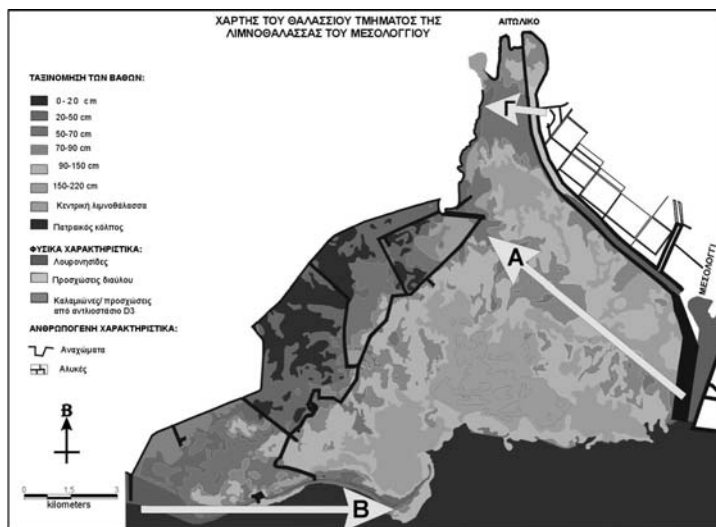
Σχήμα 5. Οι θέσεις των τριών αβαθών ζωνών που διασχίζουν την Λ/Θ του Μεσολογγίου.
