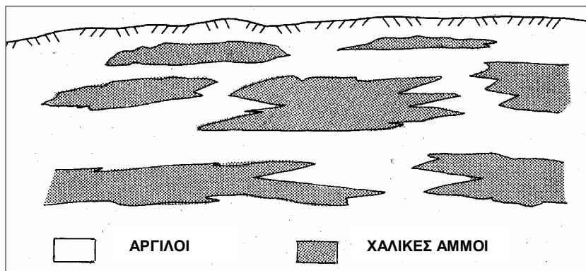
Σχήμα 2. Σκαρίφημα δομής των ιζημάτων κάτω από τη λίμνη Βιστωνίδας.
