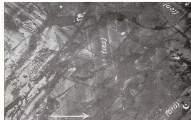
Ἔικ. 8. Τμήμα ζωνώδους κρυστάλλου σανιδίνου Σαμοθράκης εἰς τομὴν κάθετον ἐπὶ [100] ὃ βέλος κατευθύνεται πρὸς τὴν περιφέρειαν τοῦ κρυστάλλου. Αἱ ζώναι εἶναι περισσῶς διπλοθλαστικά πρὸς τὸ ἐσωτερικὸν ἢ πρὸς τὸ ἐξωτερικὸν αὐτῶν Nic. + Μεγέθ. 20X
