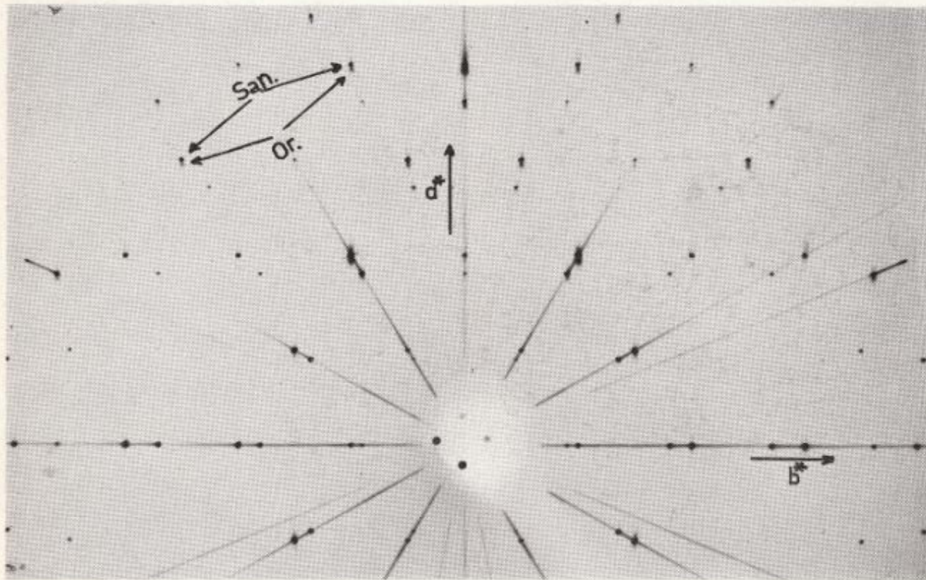
Fig. 8 Röntgenographische Precession(c)-Aufnahme von «Sanidinorthoklas» aus Hornblende-trachyandesit, Ost-Bezirjano. Parallel der a^* -Richtung unterscheiden sich deutlich die Sanidin- bzw. Orthoklas-Reflexe, während parallel b^* die Reflexe zusammenfallen. Der Kristall besteht vorwiegend aus Sanidin und nur untergeordnet aus Orthoklas. Kupferstrahlung (ungefiltert), 40 KV, 16 mamp.
